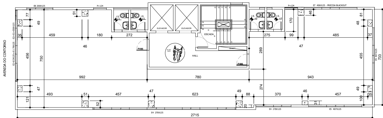
ED. MOZART - PAVTO TIPO (4°/5°/6°/7°) ESC. 1/75
