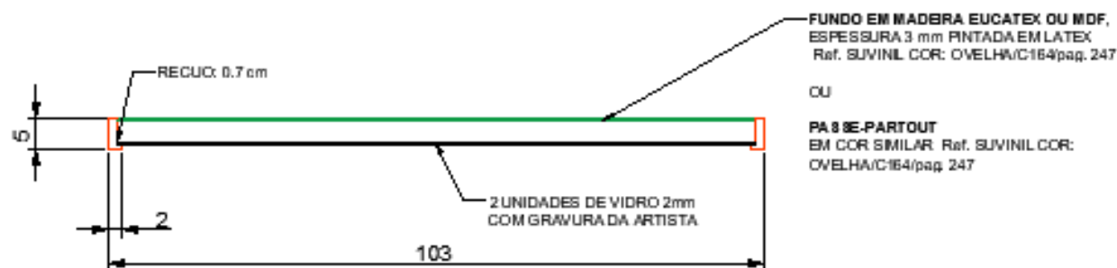
VISTA SUPERIOR - MODELO QUADRO 13º ANDAR ESCALA: 1/100 ED. SEDE
