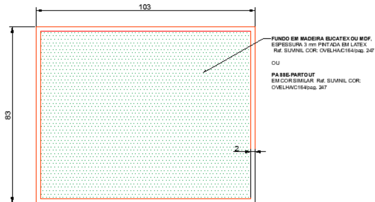
VISTA FRONTAL - MODELO QUADRO 13º ANDAR ESCALA: 1/100 ED. SEDE
