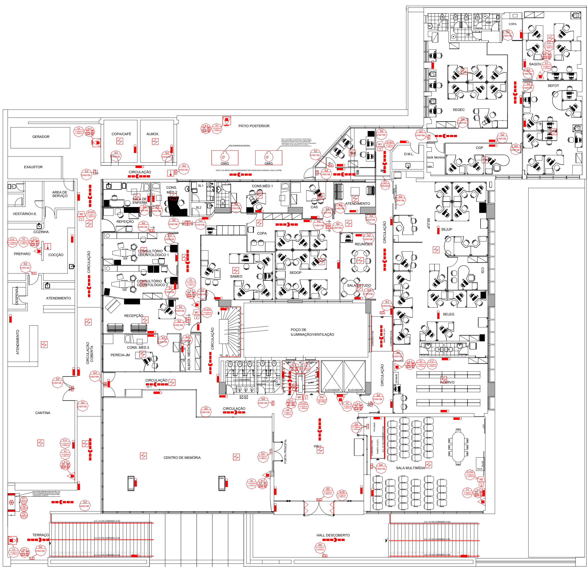
2 PLANTA BAIXA – 1º PAVIMENTO ESCALA 1:125 – 1.322,70 m²
