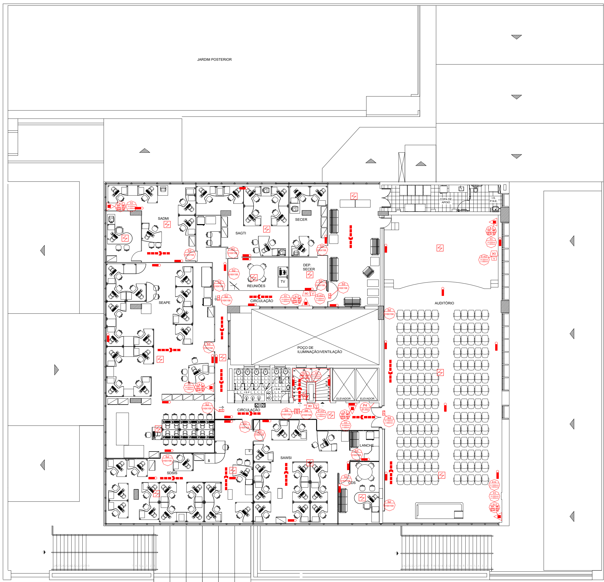
4 PLANTA BAIXA – 3º PAVIMENTO ESCALA 1:125 – 84,94 m²
