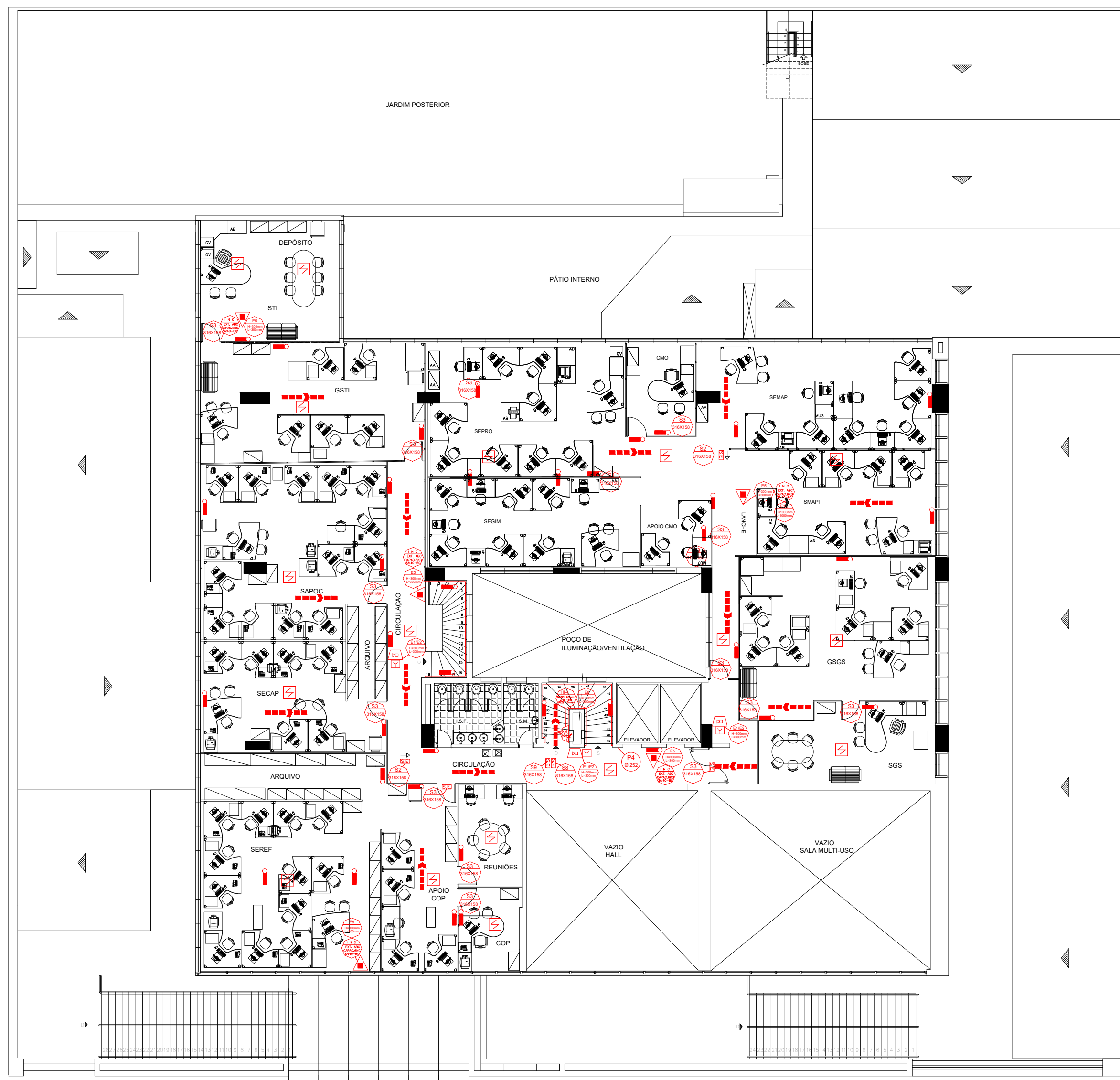
3 PLANTA BAIXA – 2º PAVIMENTO ESCALA 1:125 – 79,84 m²
