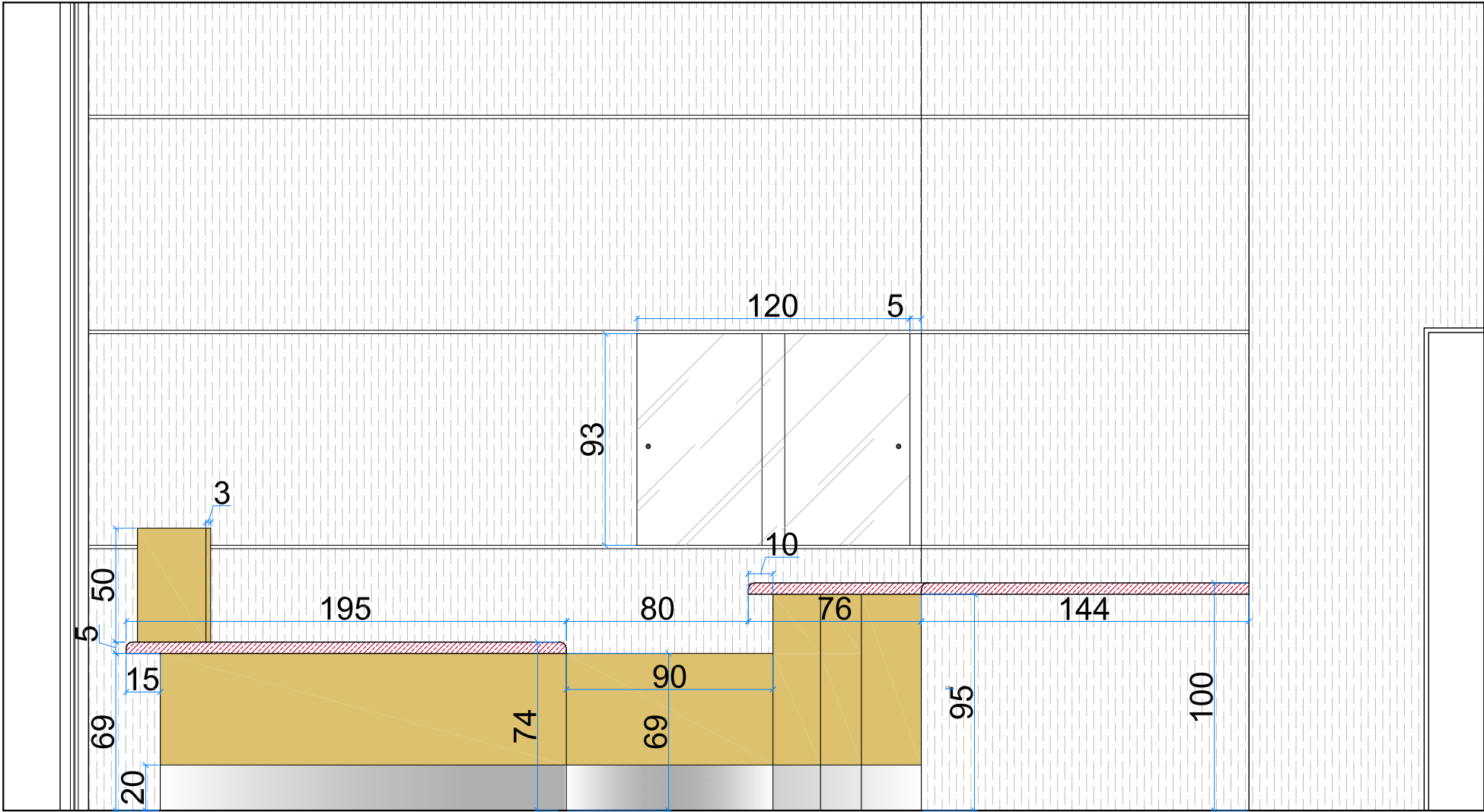
DETALHAMENTO BALCÃO ATENDIMENTO - ELEVÇÃO A ESCALA 1/30
