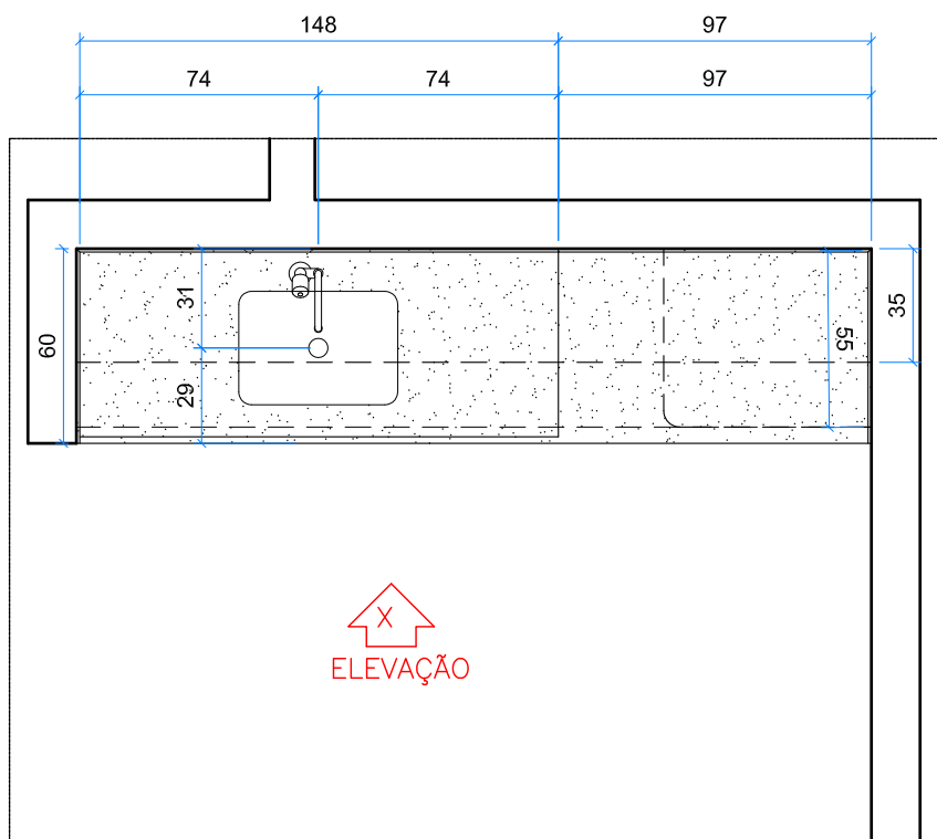
PLANTA COPA - 2º PAVTO. ESCALA 1:25
