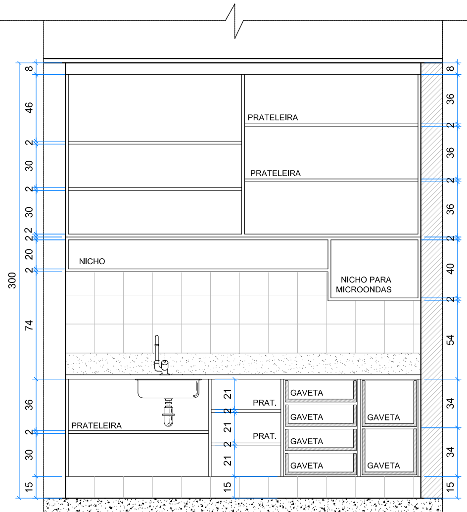
ELEVAÇÃO X - INTERNA ESCALA 1:25
