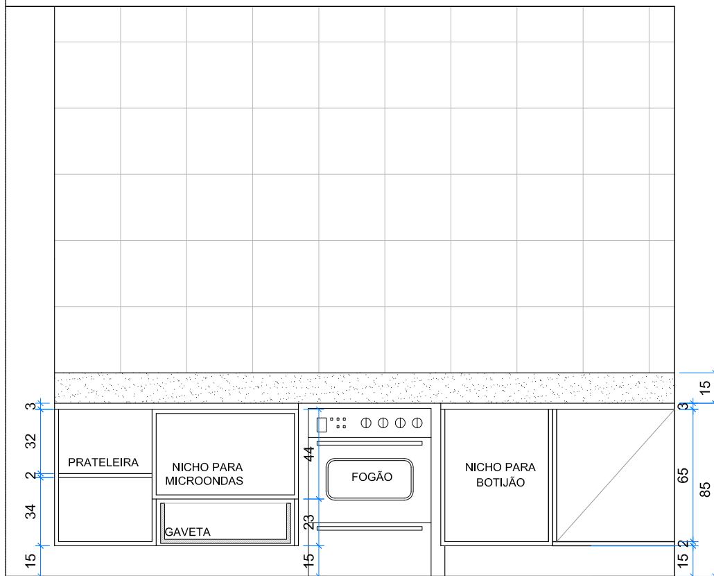
ELEVAÇÃO A - INTERNA ESCALA 1:25
