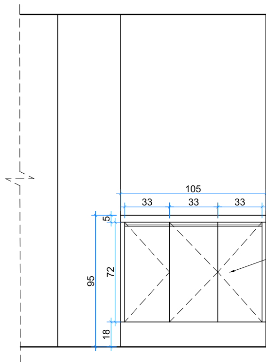
ELEVAÇÃO C EXTERNA ESC.1/25 Detalhamento armários
