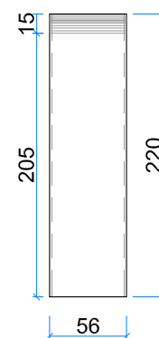
VISTA LATERAL
