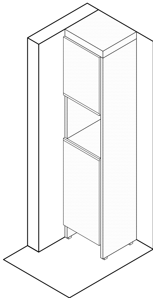
ARMÁRIO B PERSPECTIVA ESC.1/25 Detalhamento armários das copas de apoio
