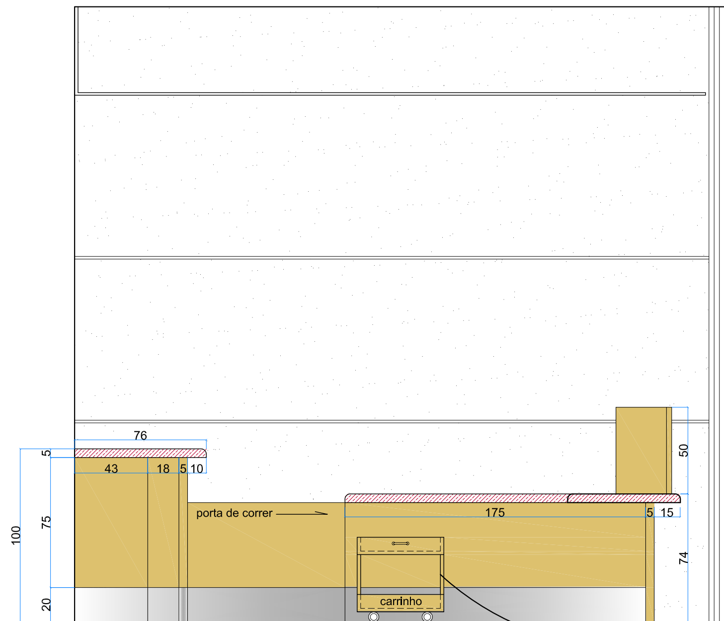
DETALHAMENTO BALCÃO ATENDIMENTO - ELEVÇÃO B ESCALA 1/30
