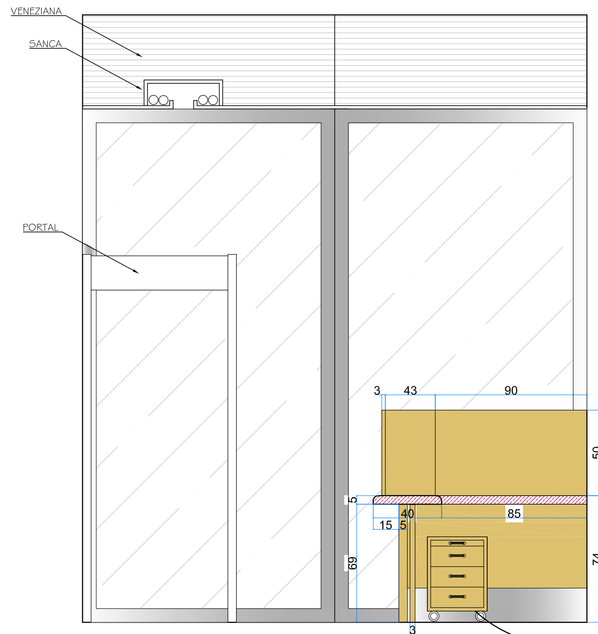
DETALHAMENTO BALCÃO ATENDIMENTO - ELEVÇÃO D
