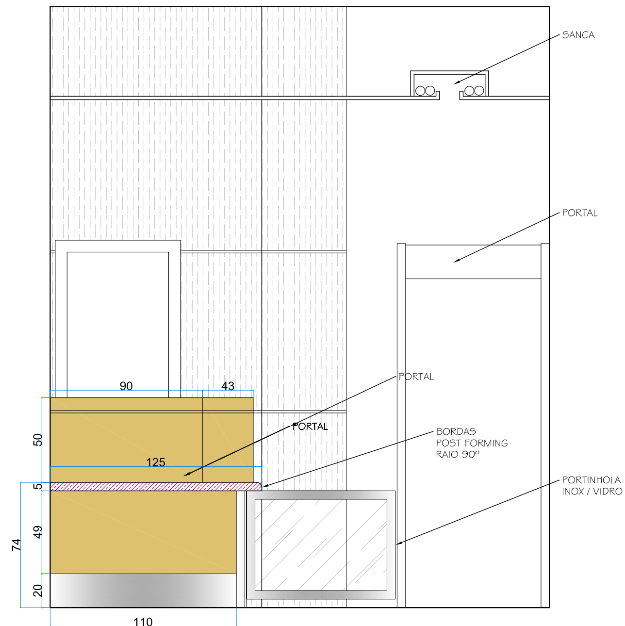
DETALHAMENTO BALCÃO ATENDIMENTO - ELEVÇÃO C
