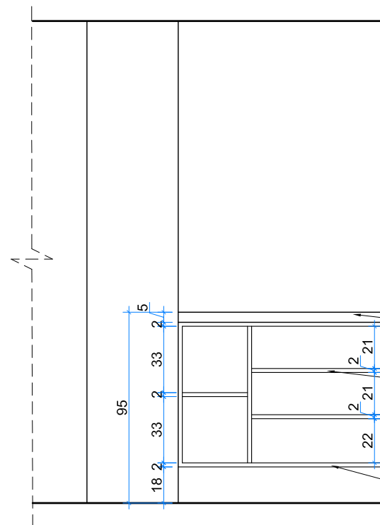
ELEVAÇÃO C INTERNA ESC.1/25 Detalhamento armários
