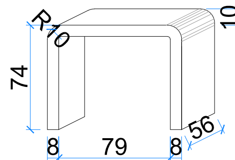
PERSPECTIVA MÓDULO B
