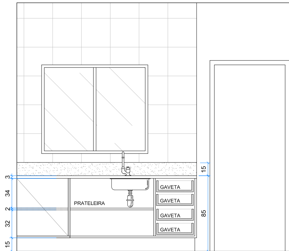
ELEVAÇÃO B - INTERNA ESCALA 1:25
