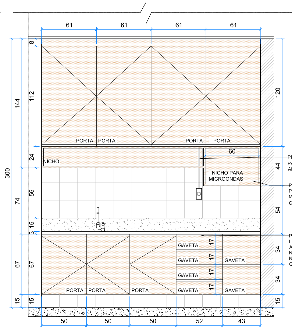
ELEVAÇÃO X - EXTERNA ESCALA 1:25
