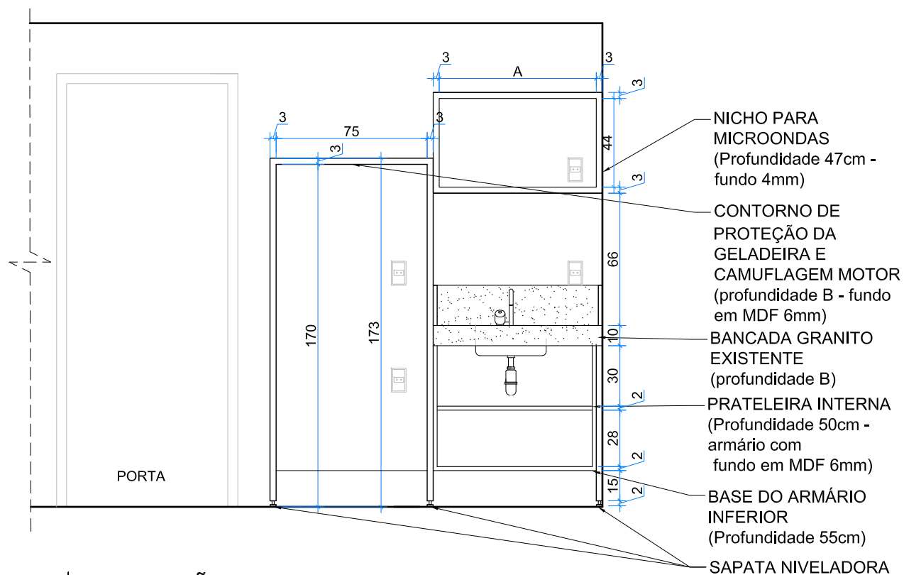
ELEVAÇÃO A INTERNA ESC.1/25 Detalhamento armários das copas de apoio
