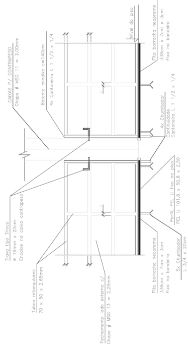
VISTA HH' ESC: 1:20
