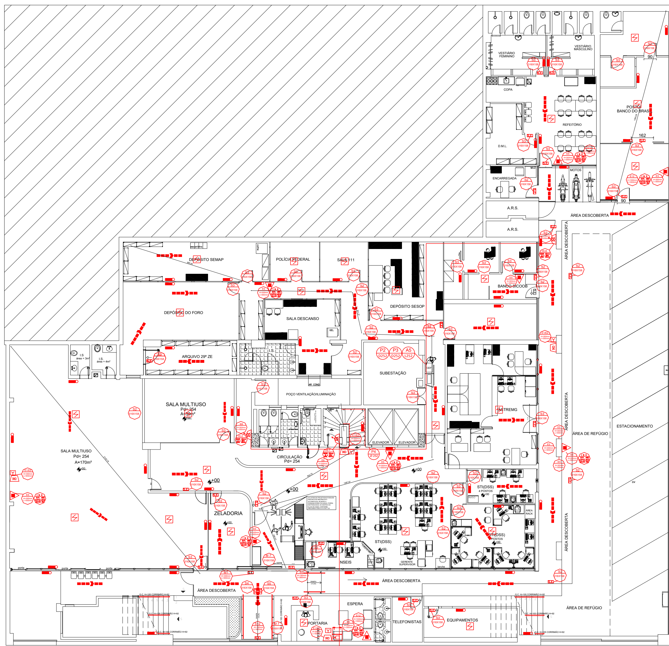
1 PLANTA BAIXA – TÉRREO ESCALA 1:125 – 143,27 m 2
