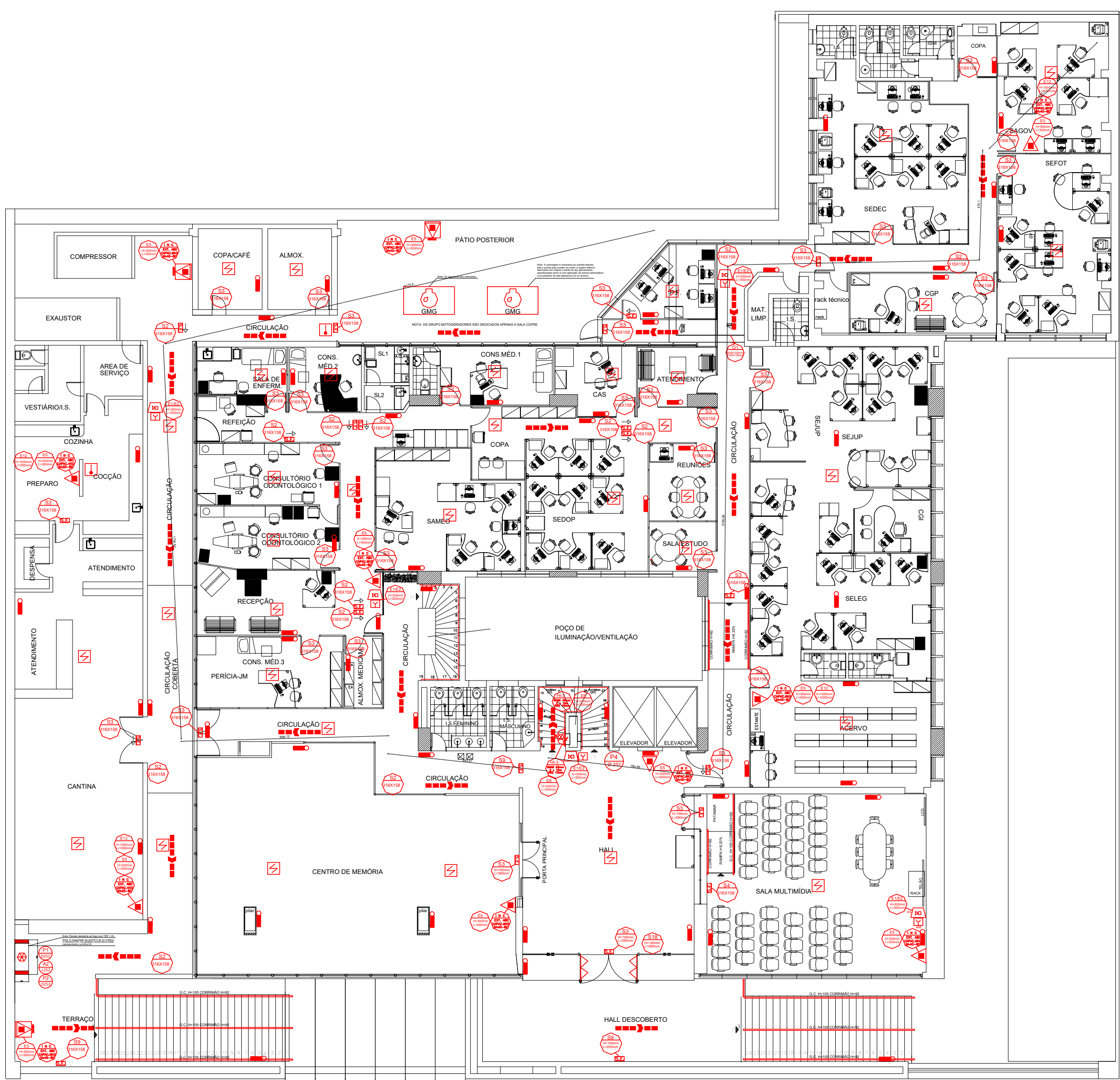
2 PLANTA BAIXA – 1º PAVIMENTO ESCALA 1:125 – 1.322,79 m 2
