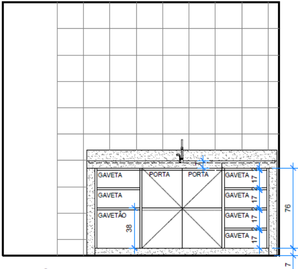
ELEVÇÃO A ESC. 1/20 ARMÁRIO SOB BANCADA
