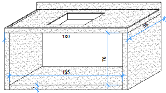
PERSPECTIVA ISOMÉTRICA BANCADA COZINHA ESC. 1/20
